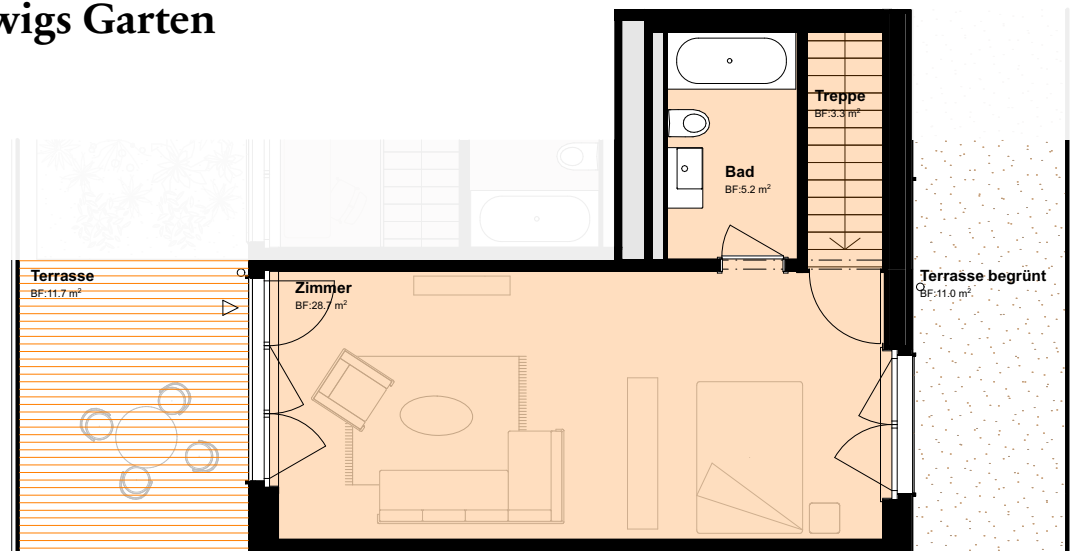
Grundriss oberes Wohngeschoss
