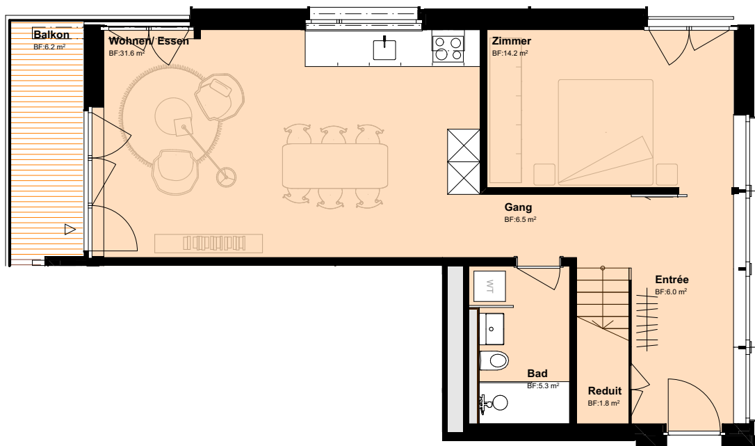
Grundriss unteres Wohngeschoss
