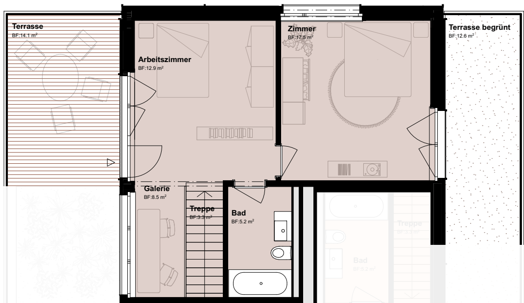
Grundriss oberes Wohngeschoss
