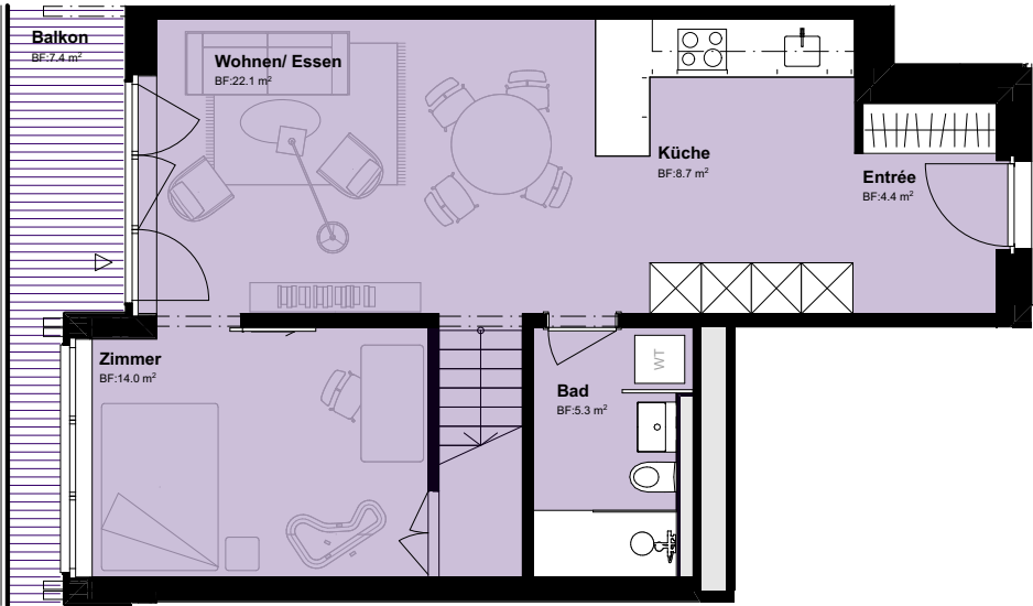
Grundriss unteres Wohngeschoss
